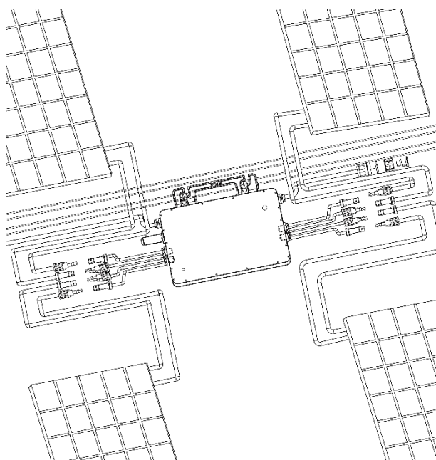
Rys.1 Pozycja montażowa mikroinwertera
